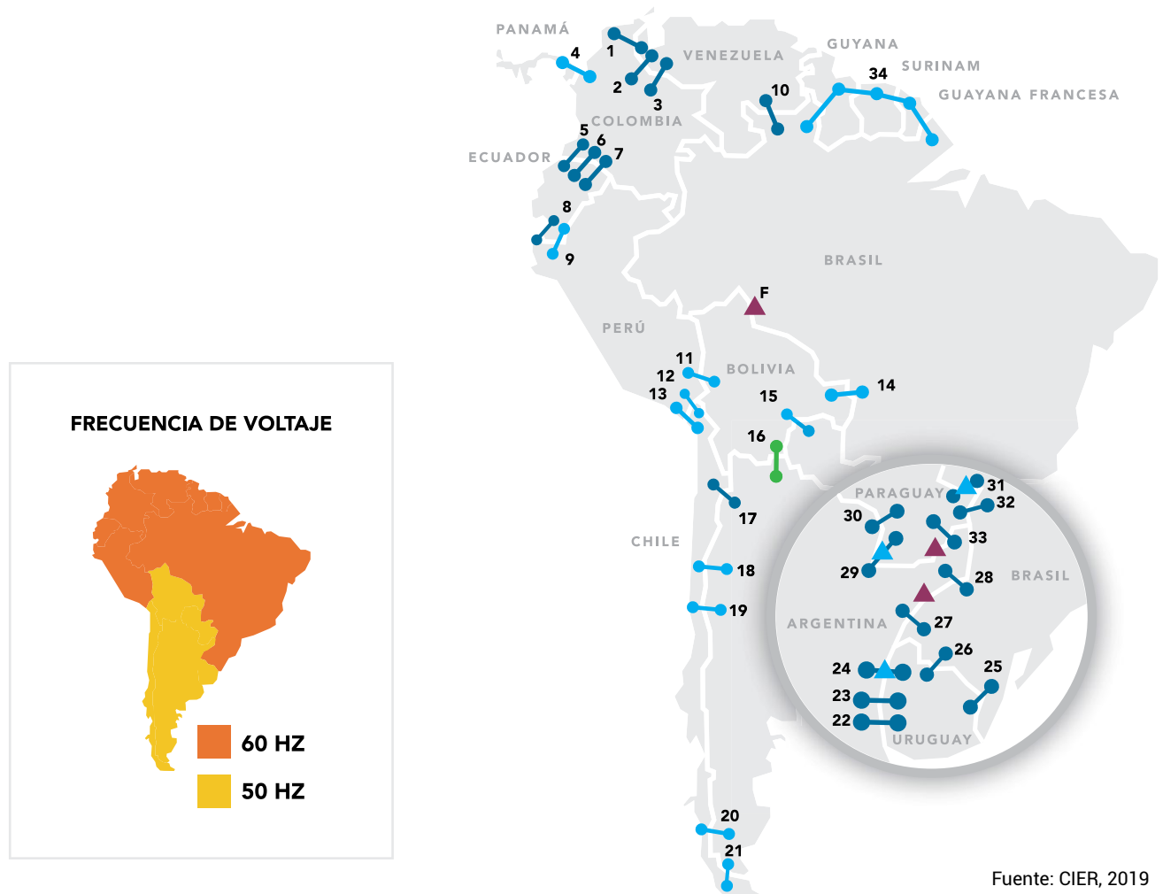
Figura 4. Vínculos de electricidad regional en Sudamérica, 2019
