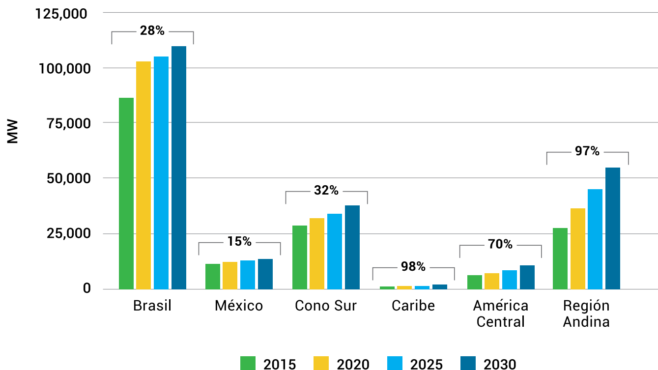
Figura 15. Proyección de instalaciones de capacidad hidroeléctrica acumulada (MW) por subregión, 2015 - 2030
